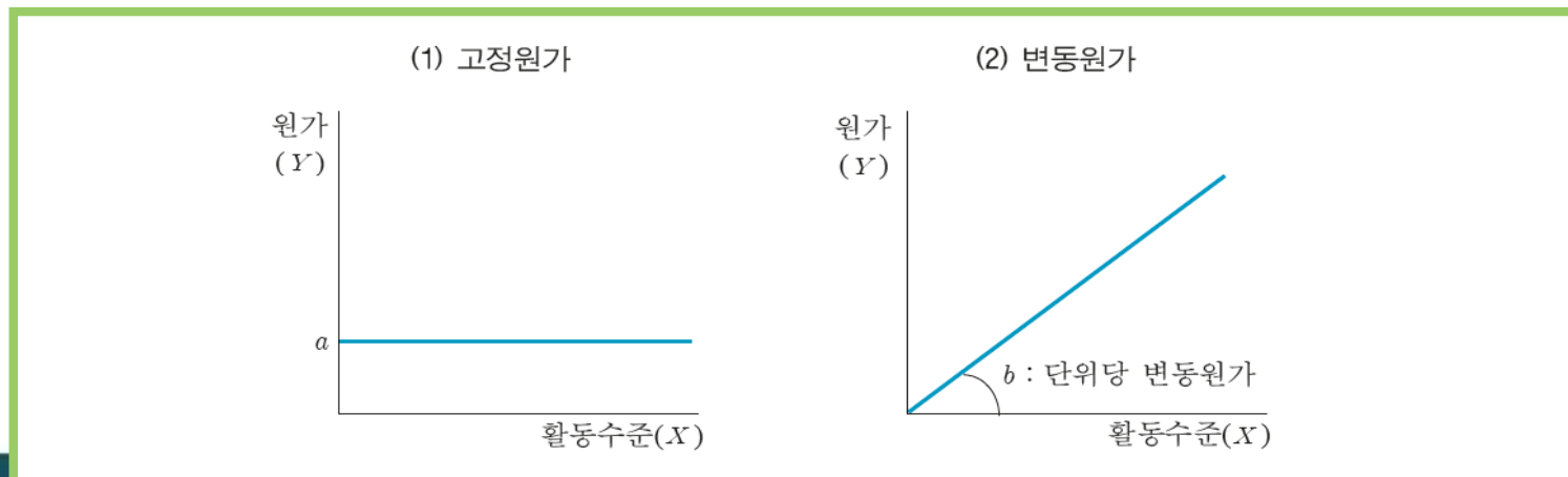
〈그림 2.5〉 원가행태
